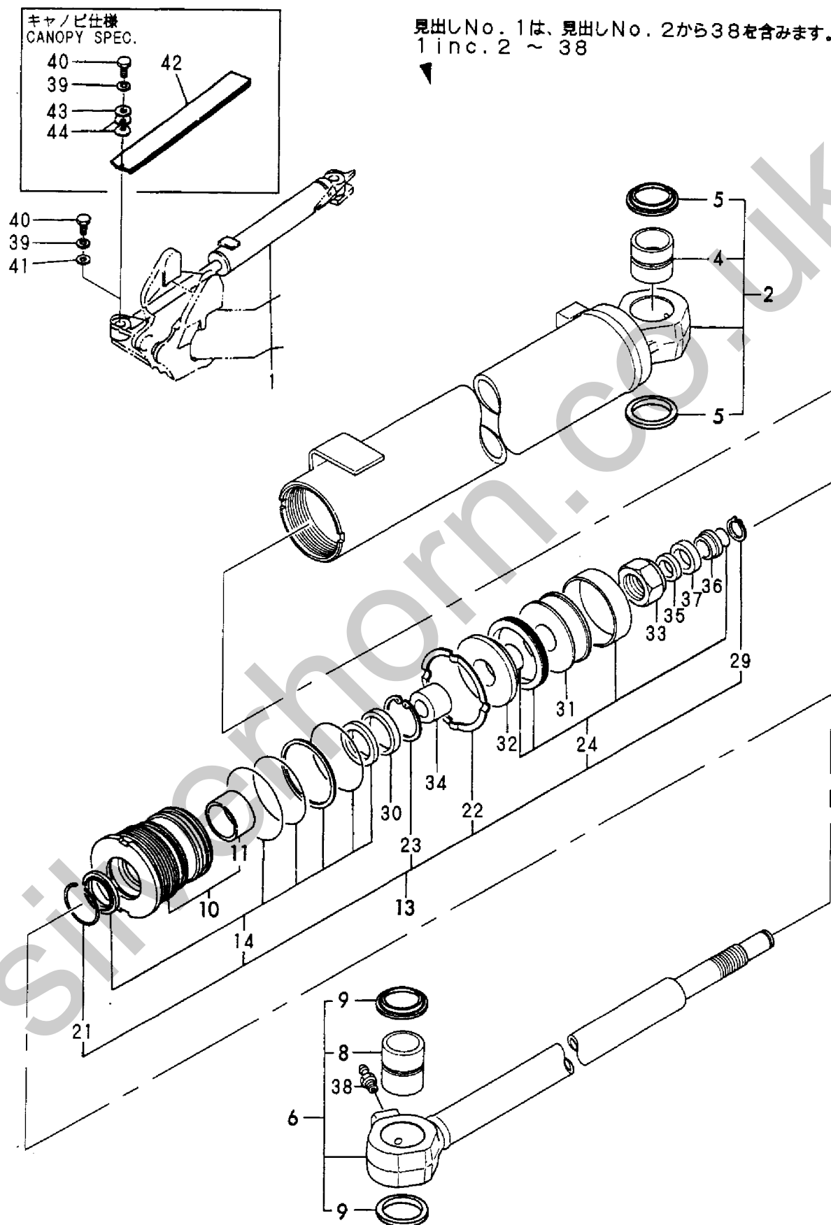
Fig. 51 スイングシリンダ SWING CYLINDER
