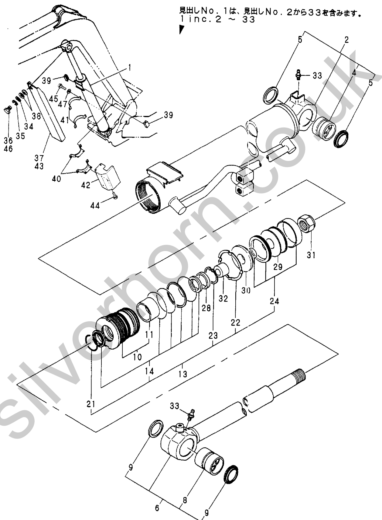
Fig. 47 ブームシリンダ (キャビン) BOOM CYLINDER (CABIN)
