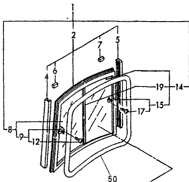
Fig. 42 キャビン (2) (サッシ) CABIN (2) (SASH)
