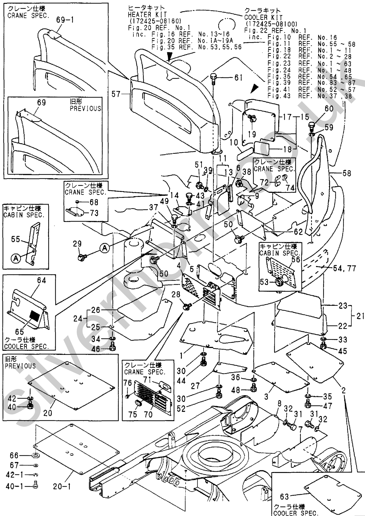
Fig. 35 フレームカバー FRAME COVER
