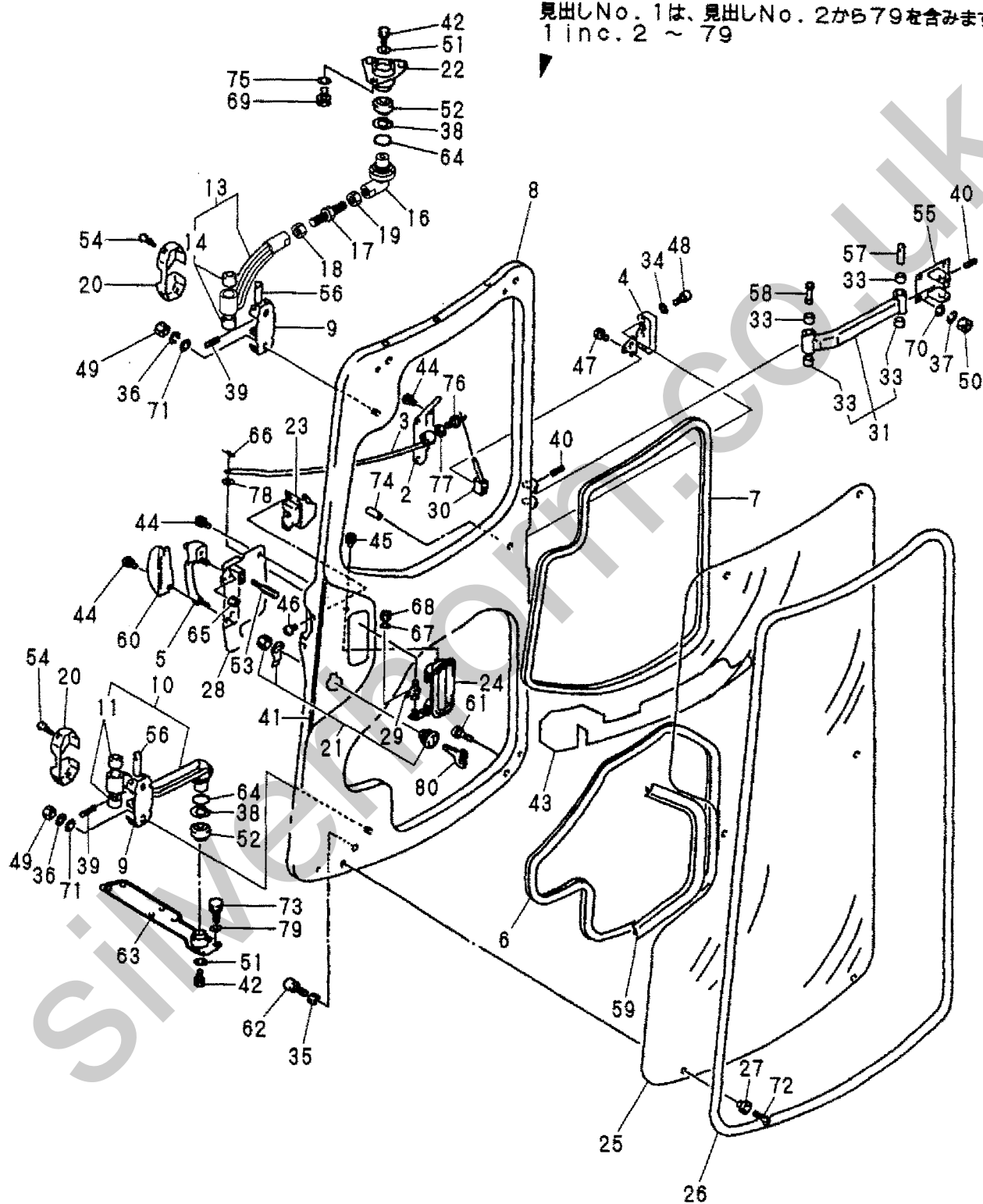
Fig. 44 キャビンドア CABIN DOOR
