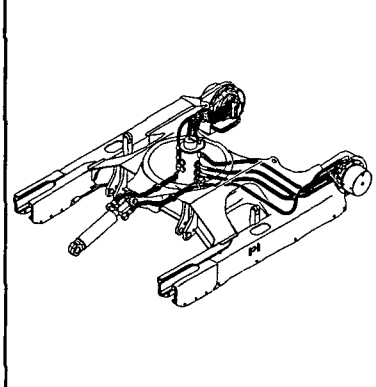
Fig. 75 油圧配管 (ブーム) HYD. OIL PIPING (BOOM)
