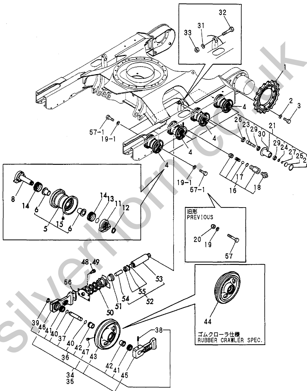
Fig. 25 ローラ&アジャスト ROLLER & ADJUST
