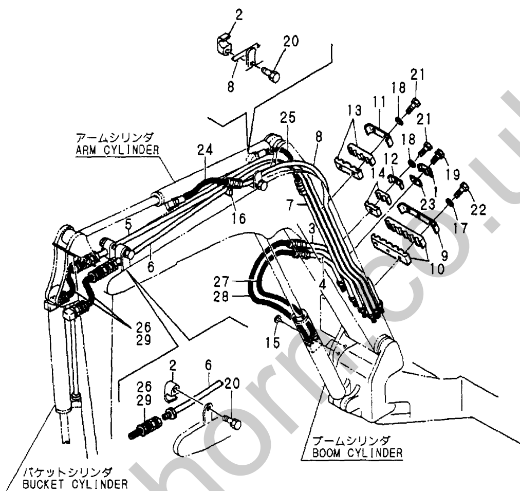
Fig. 75 油圧配管 (ブーム) HYD. OIL PIPING (BOOM)
