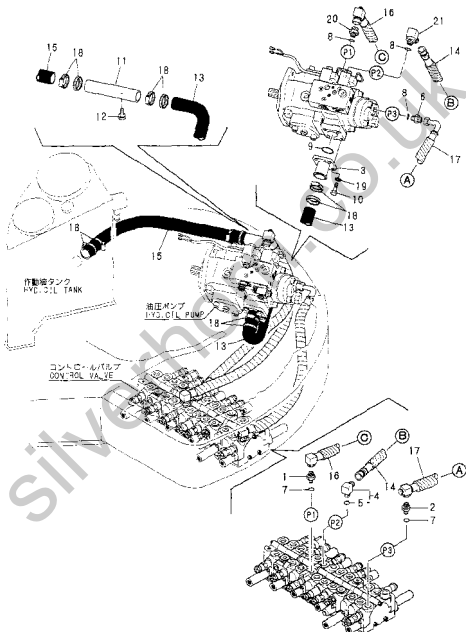
Fig. 69 油圧配管 (タンク～ポンプ～バルブ) HYD. OIL PIPING (TANK~PUMP~VALVE)
