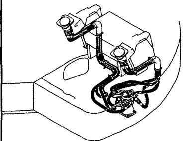
Fig. 87 コントロール配管 (4ウェイマルチチェンジ: 2) CONTROL PIPING (4 WAY MULTI CHANGE: 2)
