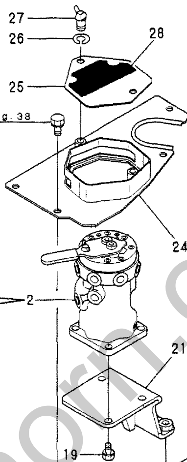
Fig. 65 ロータリバルブ (4ウェイマルチチェンジ) ROTARY VALVE (4-WAY MULTI CHANGE)
