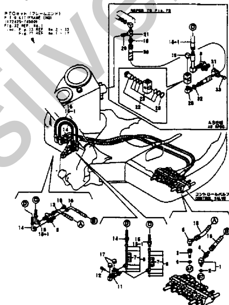
Fig. 77 油圧配管 (PTOフレームエンド) HYD. OIL PIPING (P.T.O. FRAME END)
