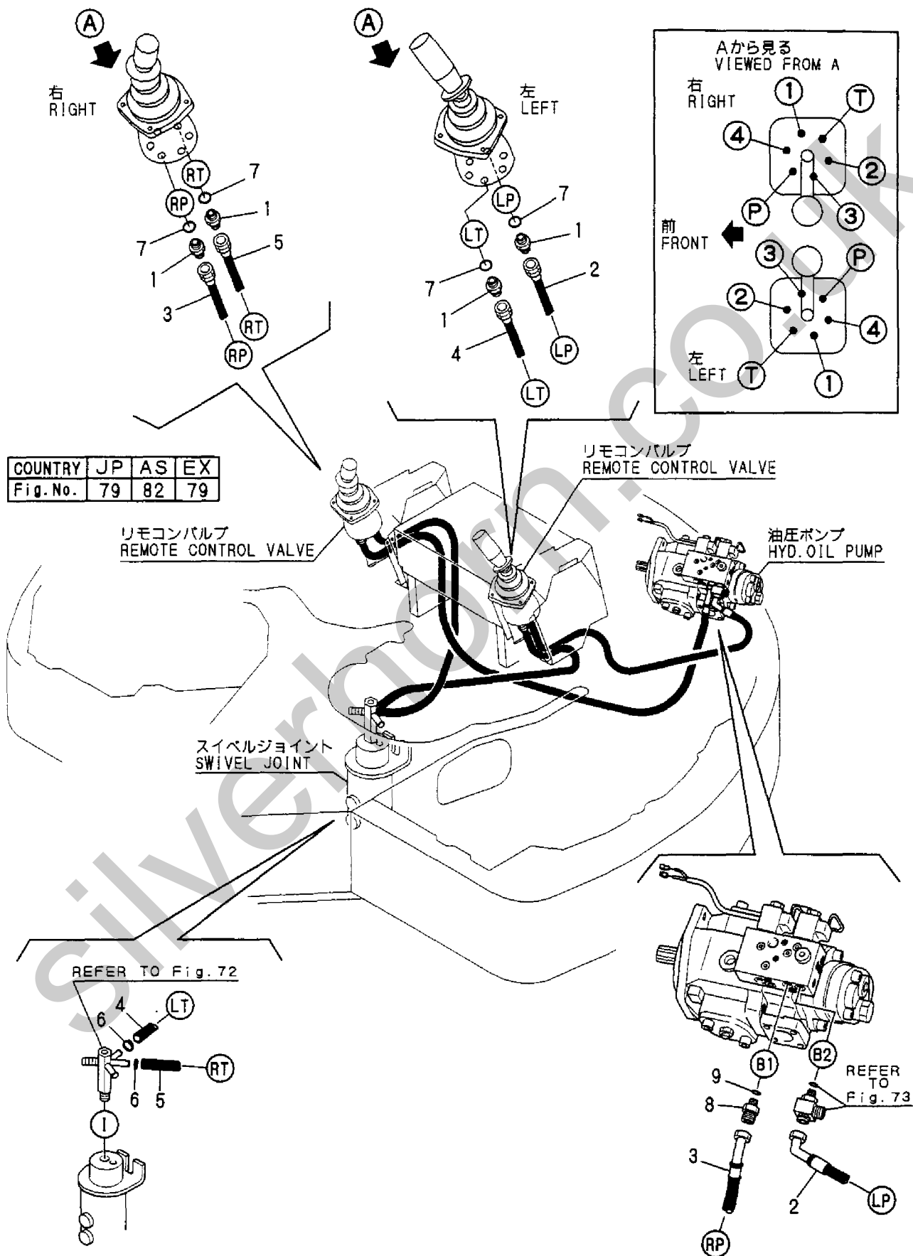
Fig. 82 コントロール配管 (ポンプ~リモコンバルブ~リターン) (AS) CONTROL PIPING (PUMP~REMO.~CON. V.~RETURN) (AS)
