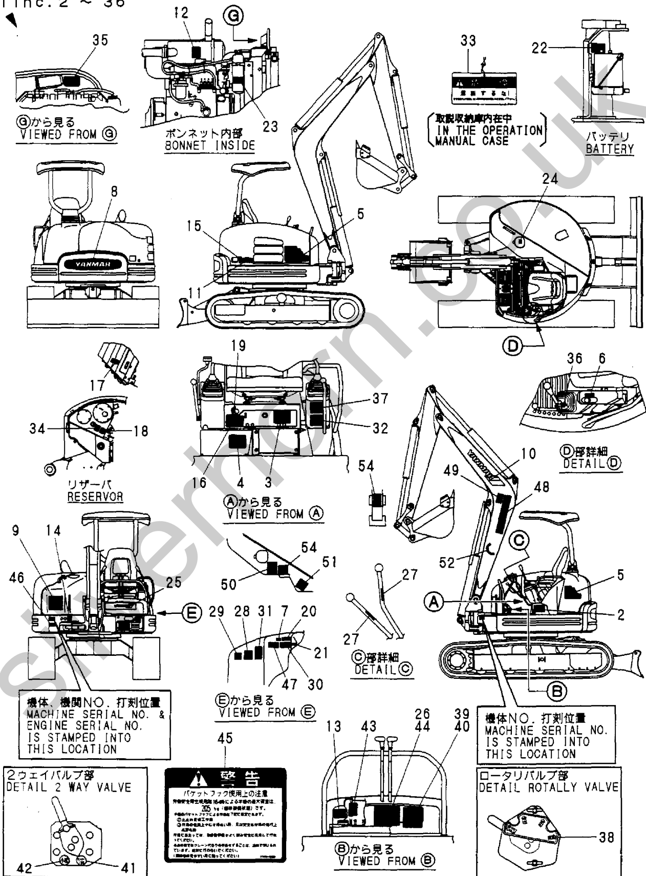
Fig. 3 銘板 (キャノピー) (JP) LABEL (CANOPY) (JP)
