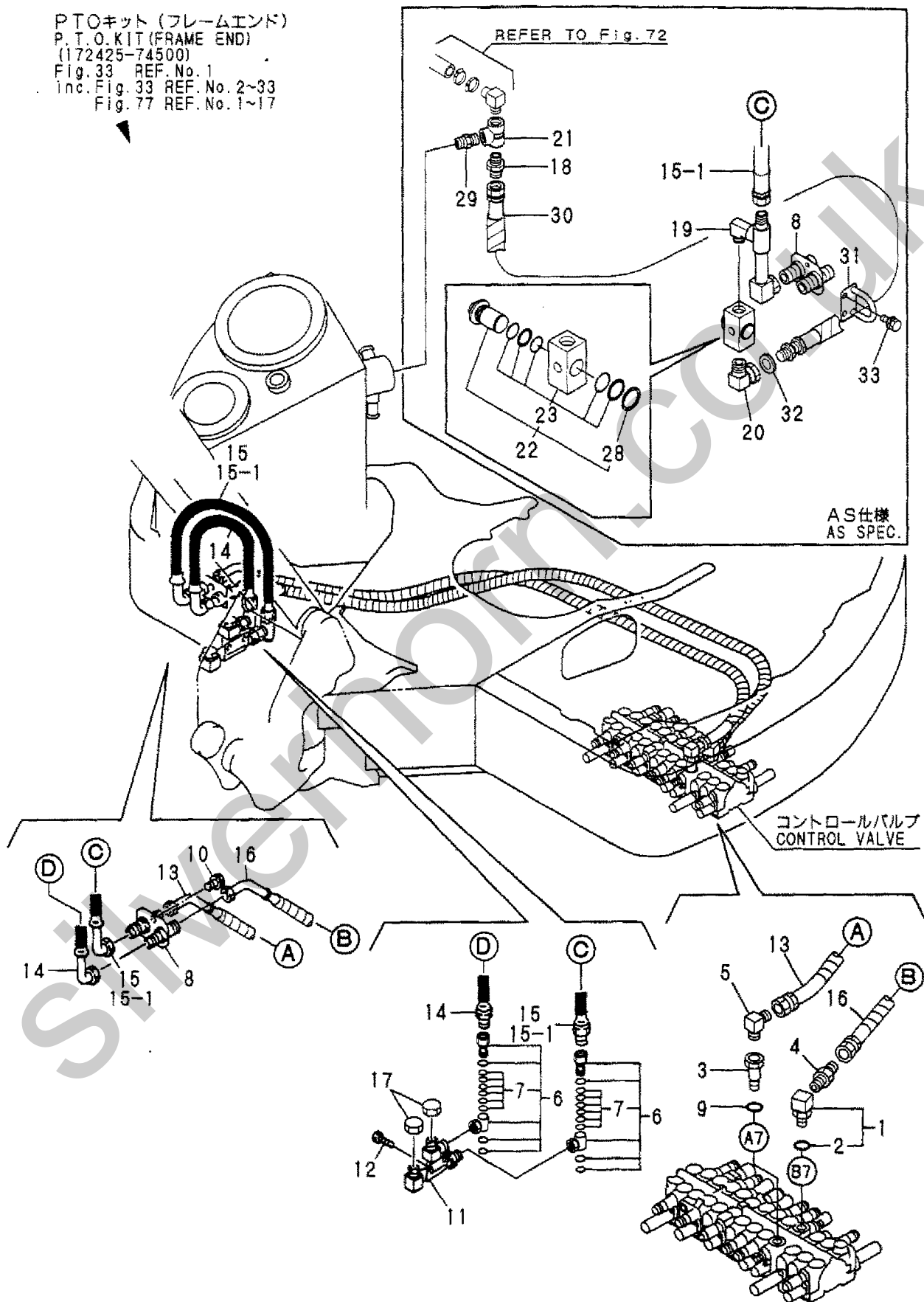
Fig. 77 油圧配管 (PTOフレームエンド) HYD. OIL PIPING (P. T. O. FRAME END)
