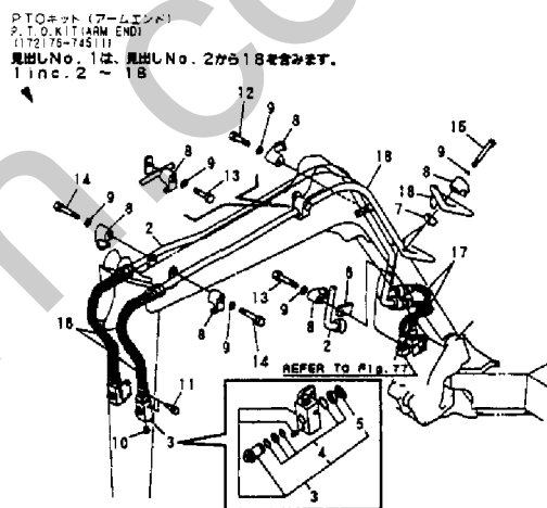
Fig. 78 油圧配管 (PTOアームエンド) HYD. OIL PIPING (P.T.O. ARM END)
