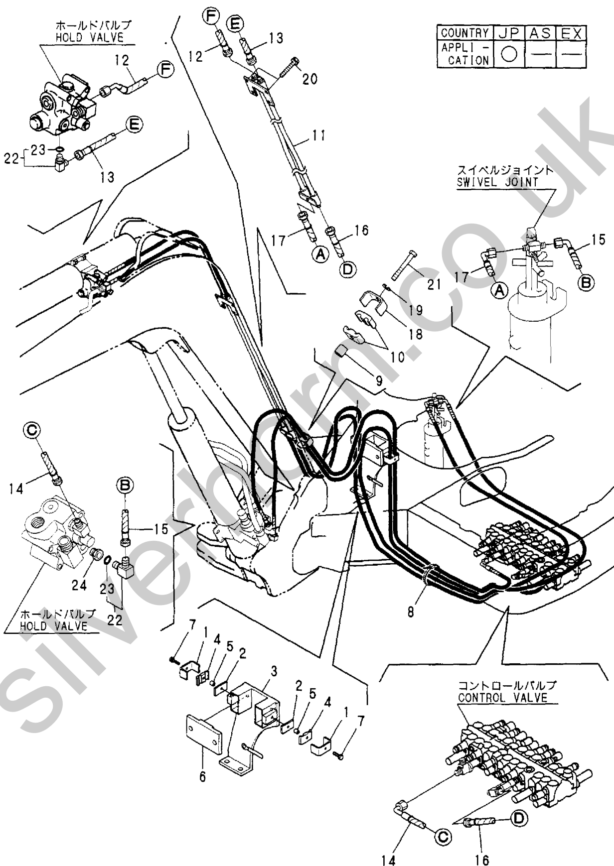
Fig. 89 コントロール配管 (ホールドバルブ) (クレーン仕様) CONTROL PIPING (HOLD VALVE) (CRANE SPEC.)
