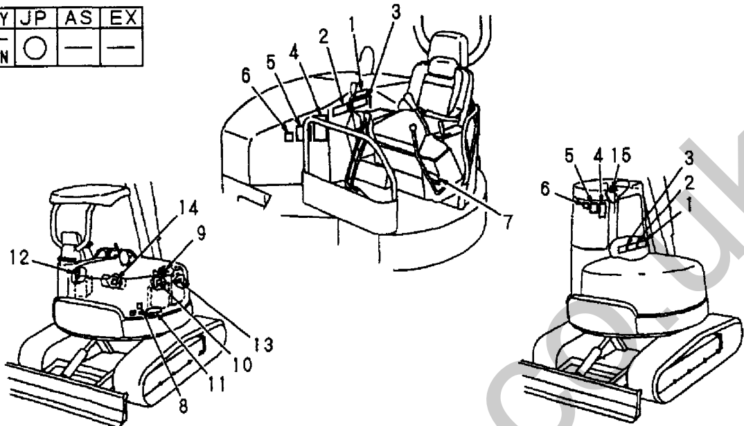
Fig. 5 安全銘板 SAFETY LABEL
