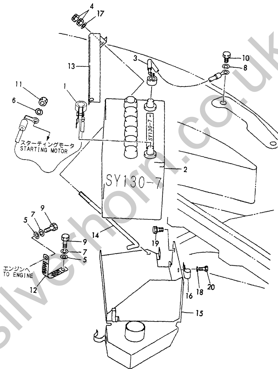
Fig. 13 バッテリー BATTERY
